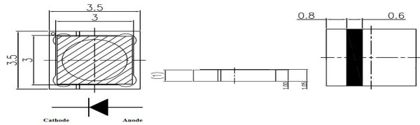
도면 및 치수 [mm]
